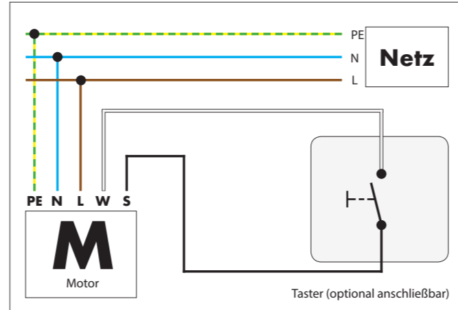
Abb.2: Anschlussschema Art. 140010 - 140050
